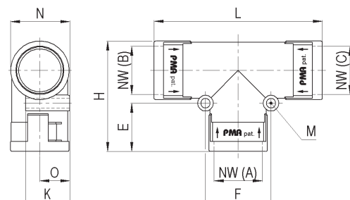
Dimensions Dimensionen
