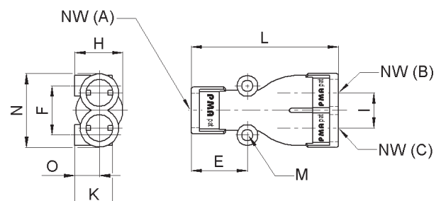
Dimensions Dimensionen
