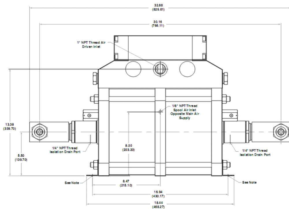
前视图
