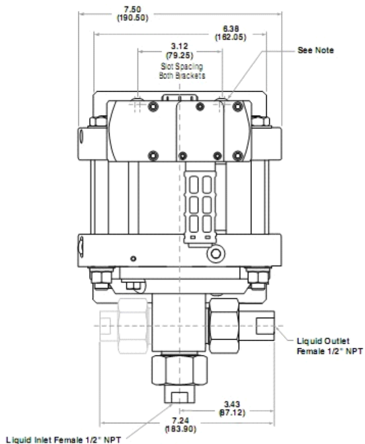
前视图
