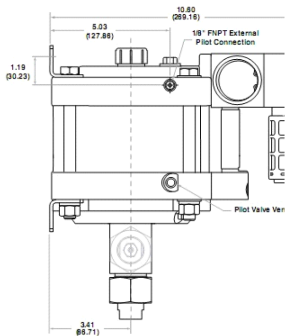
左视图
