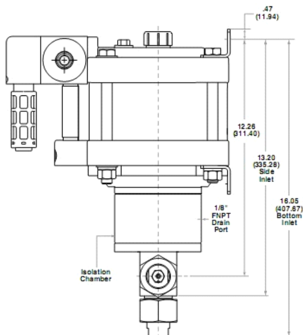
前视图
